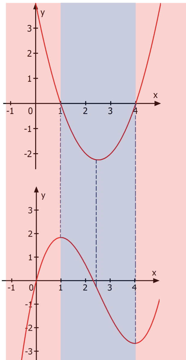
Ausgangsfunktion f(x)
